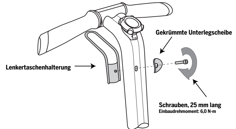
Abbildung 1. Die Lenkertaschenhalterung installieren
